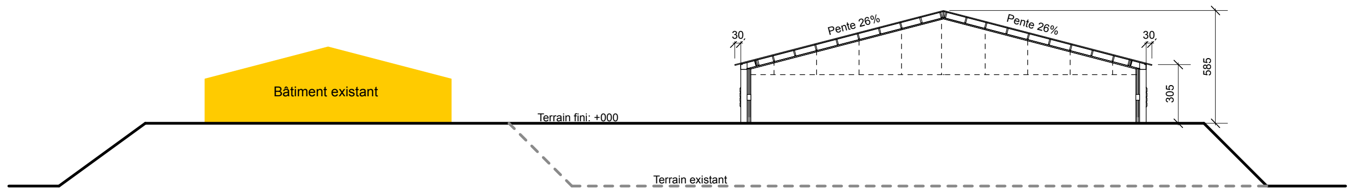
COUPE BB - 1/200e
